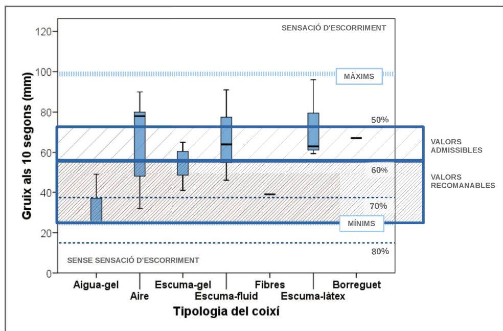
Figura 4.59. Sensació d'escorriment del coixí en funció del valor del gruix del coixí passats 10 segons
