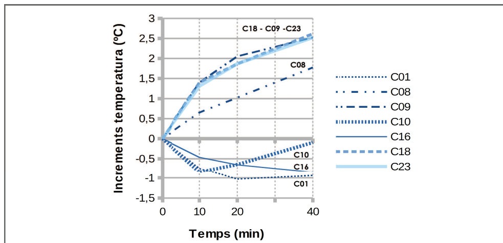
Figura 4.22. Estimació de les corbes d'escalfament per a una selecció representativa dels coixins
